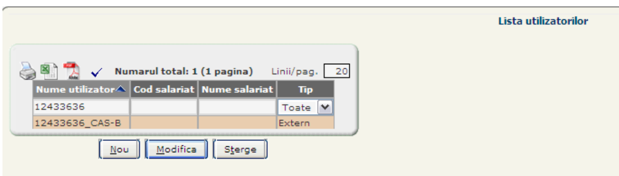
Figura 4 – Utilizator generat
